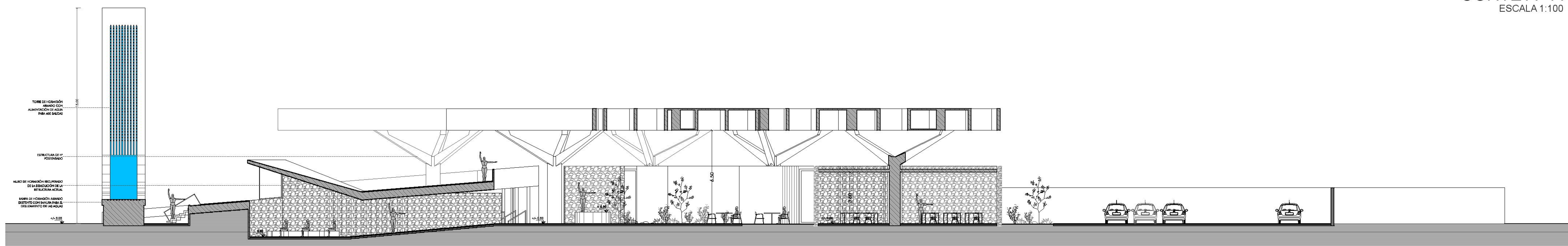
CORTE B - B ESCALA 1:100
